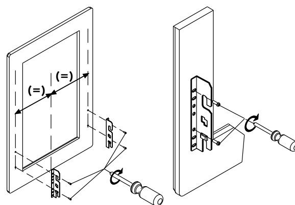
3) FISSAGGIO STAFFE SU ANTA. Fix the brackets onto the door
