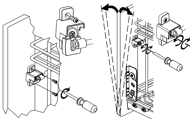
6) INSERIMENTO KIT DI REGOLAZIONE SU ANTA. Insert adjustment kit onto the door
