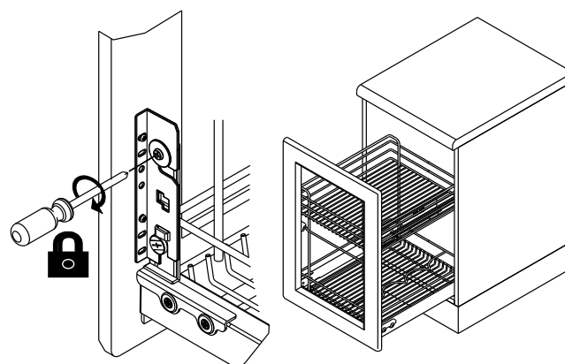
7) BLOCCAGGIO E FINE MONTAGGIO. Final tighten
